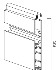
T55 ad attacco contrario in alluminio 9x55 mm
