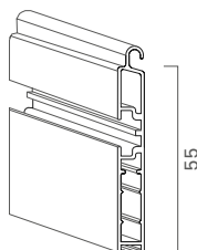
T22 ad attacco contrario in alluminio 9x55 mm
