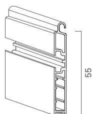
T55 ad attacco contrario in alluminio 9x55 mm
