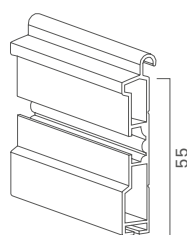
T25 ad attacco contrario in alluminio 14x55 mm
